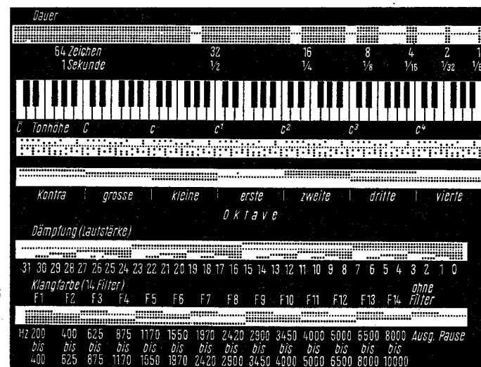
Abb. 4.9 Codierung der Parameter Zeitdauer, Frequenz, Amplitude und Spektrum auf Lochstreifen. Der waagrecht gleichmäßig durchgehende Lochabstand bildet im Verhältnis zur Lesegeschwindigkeit den «metrischen Puls» bzw. die in ein Längenmaß umgewandelte Zeiteinheit (dargestellt nach Informationsbericht Siemens-Studio, München 1962).
