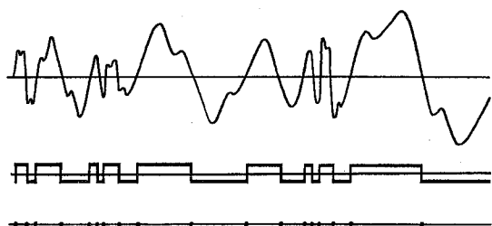
Abb. 3.19 Schematisierte Kurve eines Sprechsignales (oben) und dieselbe Kurve nach Amplitudenbeschneidung mittels eines Schmitt-Triggers (Mitte). Erhalten bleibt die zeitliche Ordnung der Nulldurchgänge (unten).
