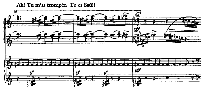
Abb. 3.27 Giuseppe Verdi: Otello, 4. Akt 1. Szene (oben); Arthur Honegger: Le roi David, No 12 Incantation (unten).
