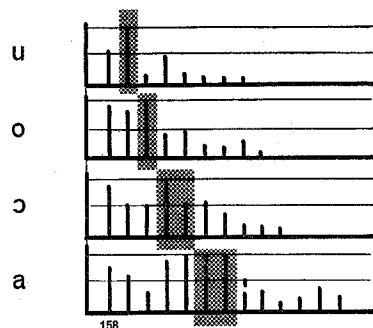
Abb. 3.9 Wechsel der Vokalklangfarbe. Durch Amplitudenmodulation der harmonischen Teiltöne kann die männliche Stimme ohne Veränderung des Grundtones bequem von einer Vokalfarbe in jede andere übergehen.
