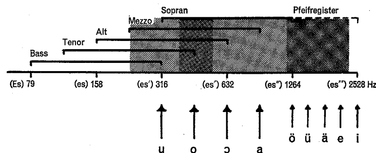
Abb. 3.8 Vokalformantbereiche und ungefährer Tonhöhenumfang der menschlichen Gesangstimmen.
