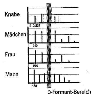
Abb. 3.4 Das harmonische Spektrum des Vokales ɔ (sehr dunkler, gegen das offene o getönter a-Vokal). Es ist gekennzeichnet durch einen ɔ-Formanten im absoluten Frequenzbereich von etwa 600 bis 650 Hz.
