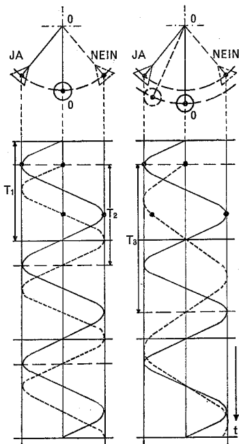
Abb. 2.12 Zwei Pendel gleicher Länge schwingen mit derselben Periodenzeit bzw. Frequenz ( T_1 = T_2 ); auch wenn ihre Schwingungen gegeneinander verschoben sind, bleibt daher die Verschiebung immer dieselbe (links). Zwei Pendel ungleicher Länge dagegen schwingen nicht mit derselben Periodenzeit bzw. Frequenz ( T_1 \neq T_2 ); daher verschieben sich die Phasen ihrer Schwingungen (rechts).
