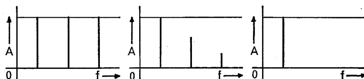
Abb. 2.8 zeigt die Spektren eines aus drei Sinustönen gebildeten Akkordes (links), der durch Verringerung der Amplituden zweier Sinustöne in einen Klang (Mitte) und schließlich in einen einzigen Sinuston übergeführt wird (rechts).
