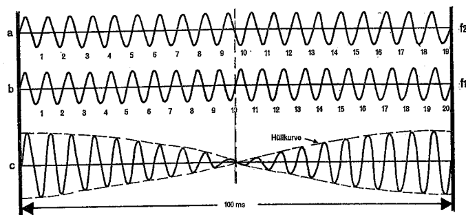
Abb. 2.13 Zustandekommen einer Schwebung (c) durch allmähliche Phasenverschiebung zweier überlagerter Sinusschwingungen verschiedener Frequenz (a und b). Im Augenblick völliger Phasengleichheit beider Sinusschwingungen erreicht die Hüllkurve der Schwebung ihre maximale (links und rechts) und bei entgegengesetzter Phase ihre minimale Amplitude (Mitte). Vgl. Photo 23.
