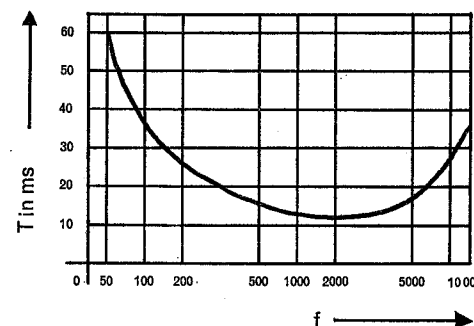
Abb. 2.20 Kurve der erforderlichen Minimalzeit zur Erregung einer diskreten Tonhöhenempfindung im menschlichen Ohr. Für ein Sinussignal von 1000 Hz liegt dieser Zeitwert etwa bei 12 ms; es braucht also ungefähr 12 Perioden, damit ein Sinussignal mit der Frequenz f = 1000 Hz vom Ohr als Tonhöhe erfaßt werden kann. 3 bis 4 Perioden sind notwendig für ein Signal von 200 Hz, ungefähr 250 für ein solches von 10 kHz (Darstellung nach Stevens und Davis).
