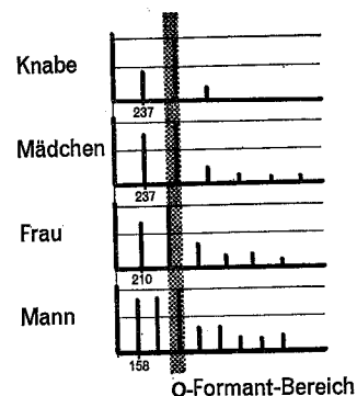
Abb. 3.3 Das harmonische Spektrum des Vokales o zeigt verschiedene Amplituden-Frequenz-Verhältnisse, je nachdem ob der Vokal von einem Mann, einer Frau, einem 8jährigen Mädchen oder einem 4jährigen Knaben gesprochen wird. Gemeinsam ist jedoch allen diesen Spektren ein o-Formant im absoluten Frequenzbereich zwischen etwa 420 und 480 Hz. Die Zahlenangaben unterhalb der ersten Harmonischen bedeuten im folgenden stets die Grundtonhöhe in Hz.
